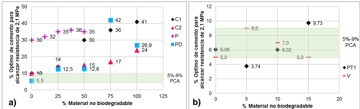
Figura 3. Porcentaje cemento óptimo, suelo A-2. a) por sustitución. b) por adición
