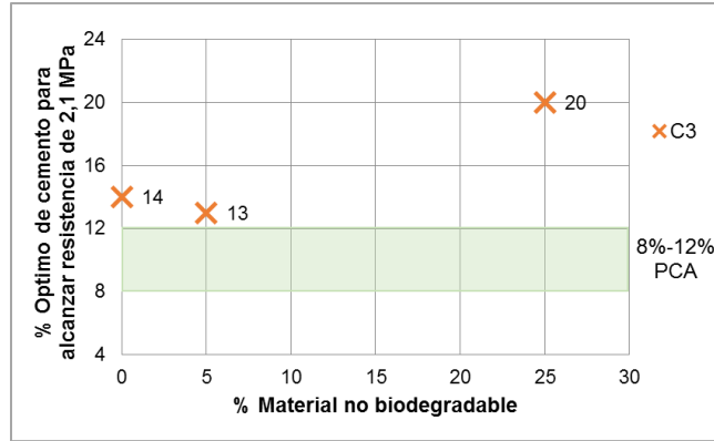
Figura 4. Porcentaje cemento óptimo, suelo A-4 por adición.
