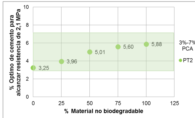
Figura 2. Porcentaje óptimo de cemento, suelo A-1-a por sustitución.
