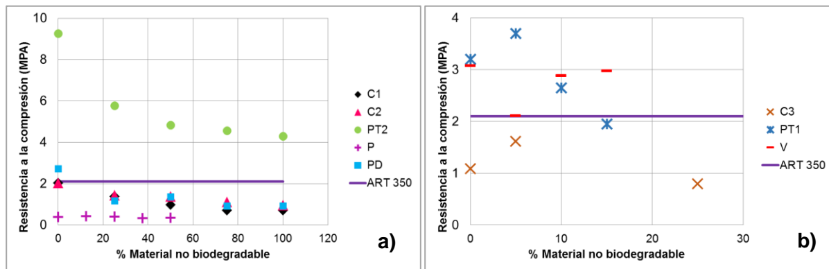
Figura 1. Comparación resistencia a la compresión suelos. a) por sustitución. b) por adición.
