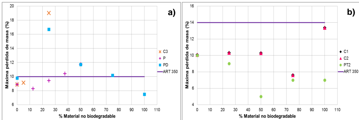
Figura 5. Máxima pérdida de masa de la mezcla compactada en prueba de humedecimiento y secado. a) Suelos A-2-6 y A-4. b) Suelos A-1-a y A-2-4
