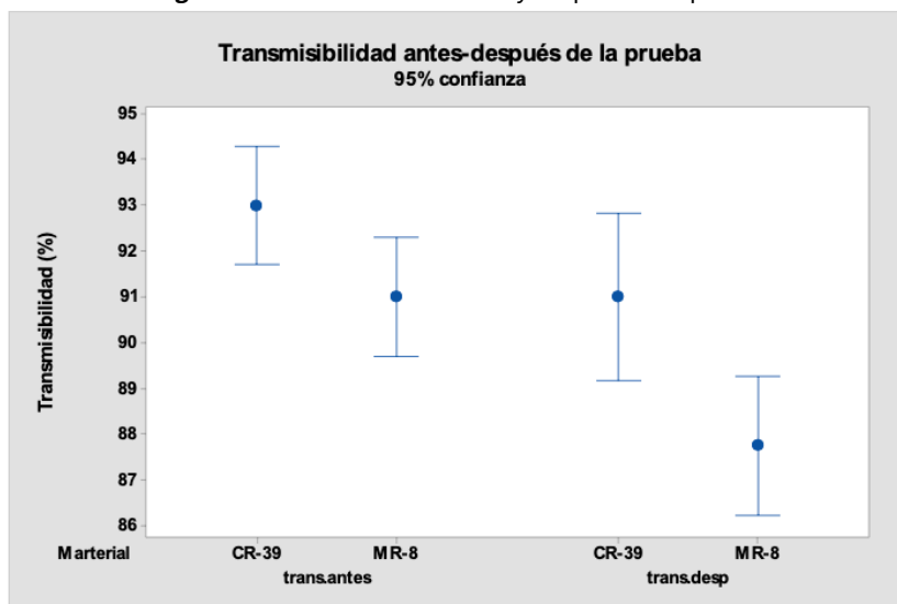
Figura 2. Transmisibilidad antes y después de la prueba
