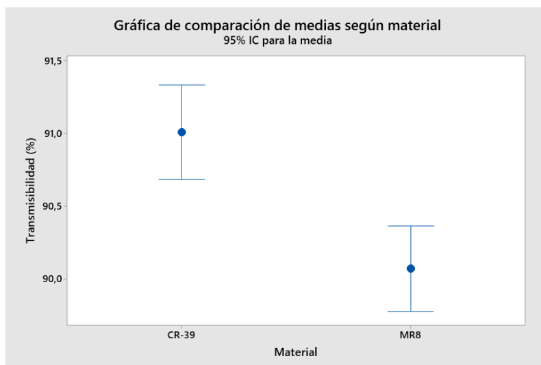
Figura 1. Comparación de medias según material, con respecto a las mediciones a 535 nm, luz visible
